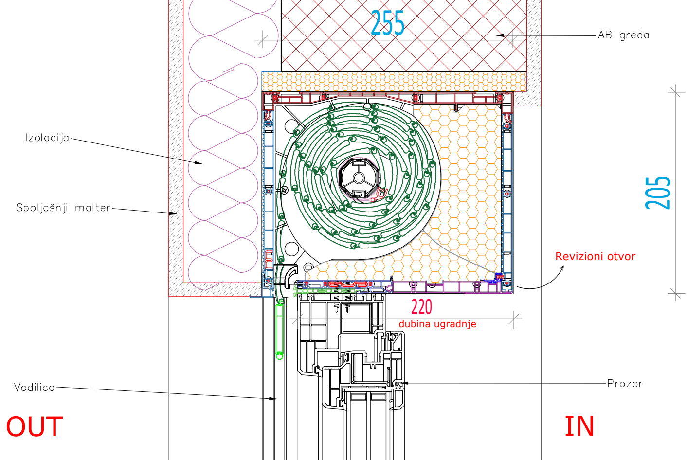
PVC vodilica ravna MINI 60x35 - bez komarnika
