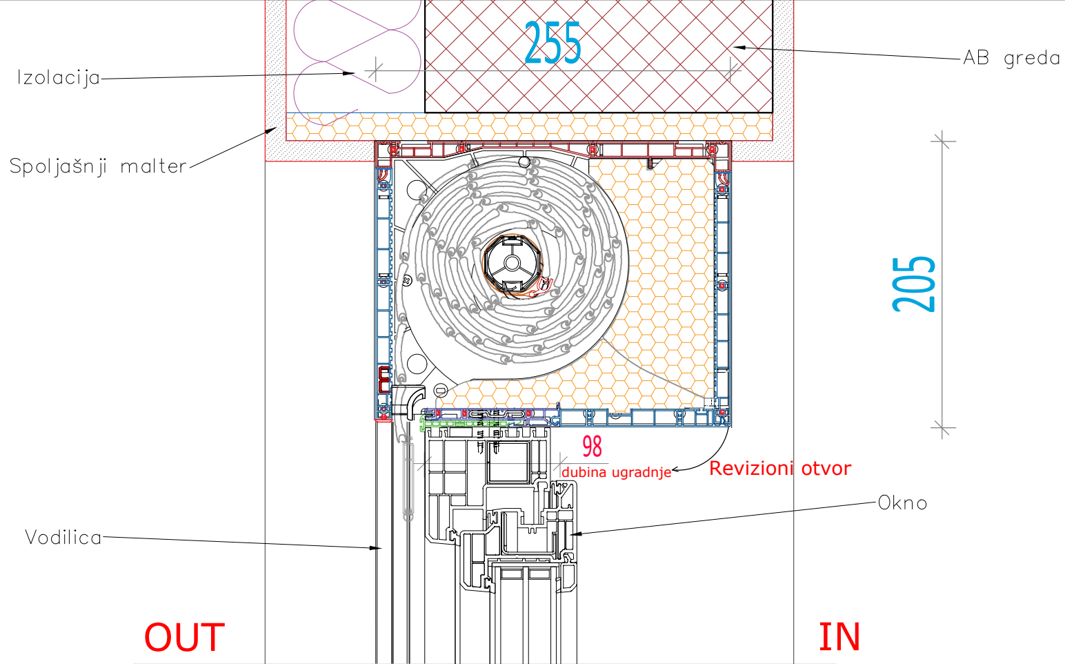
PVC vodilica ravna MINI 60x35 - bez komarnika
