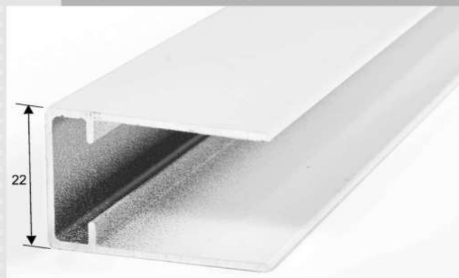
Gornja vodilica reverzibilnog smart komarnika
