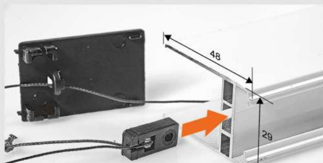
jedini način provlačenja i fiksiranja konca za vodilicu
