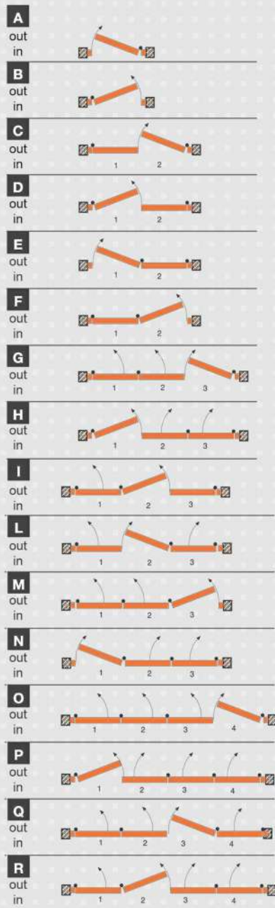
Plastična šarka sa oprugom
