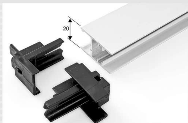
Fiksni profil reverzibilnog komarnika sa levim i desnim čepom
